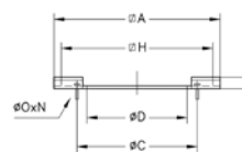
PA. Placa de adaptación para montaje de accesorios, en extractores de tejado
