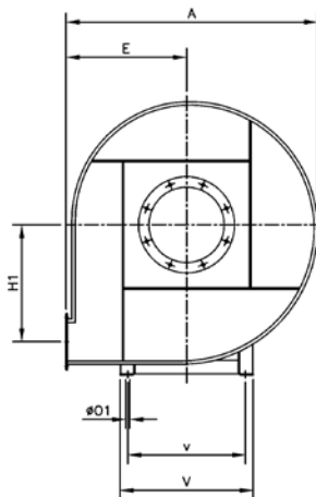
Boca de aspiración
