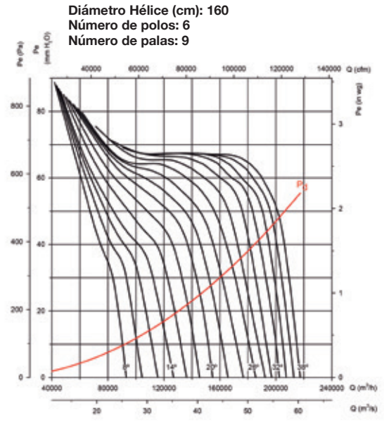
Potencia absorbida
