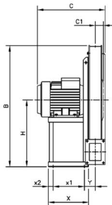
Boca de impulsión CAS-680/790
