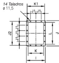
Boca de impulsión CAS-1250-2T-15/A CAS-1456-2T-25/A CAS-1663-2T-50/A
