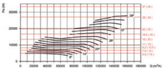
Potencia absorbida
